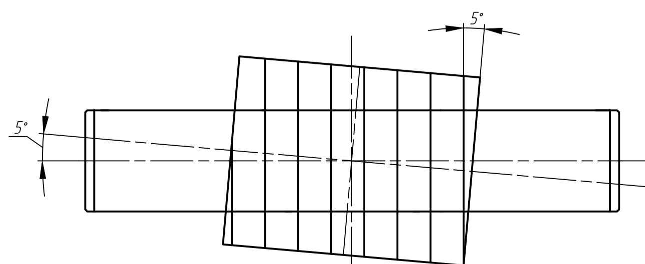
Схема установки червячной фрезы
