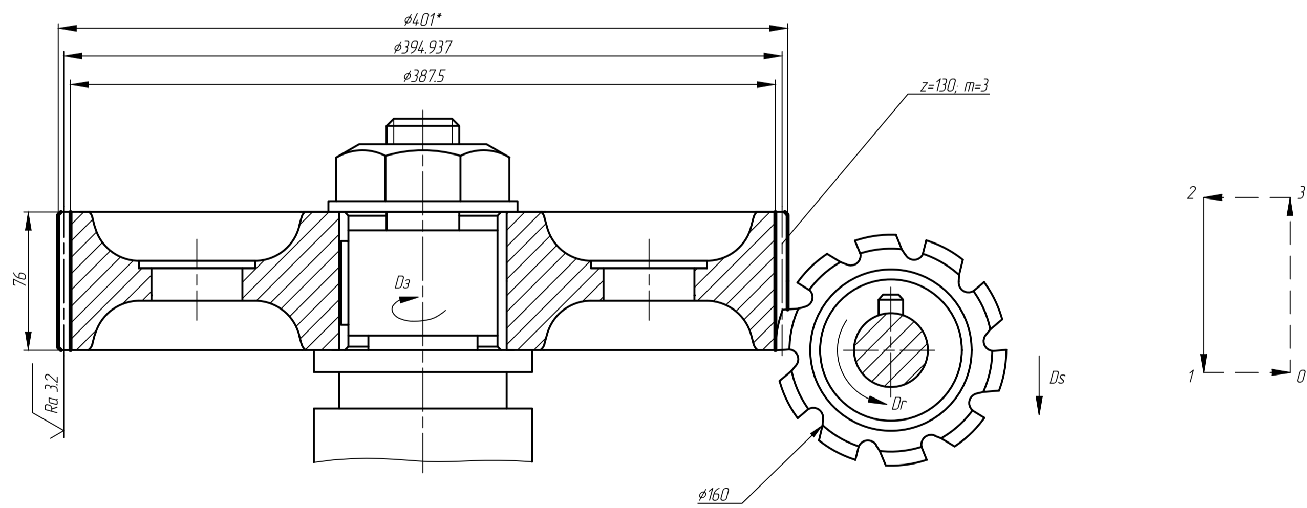
Схема установки червячной фрезы
