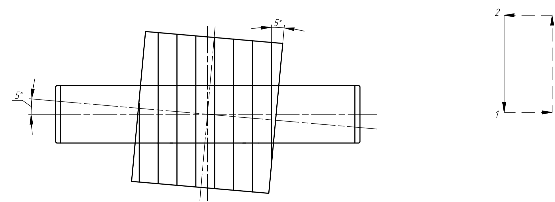
Схема установки червячного круга
